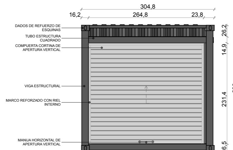
ALZADO
