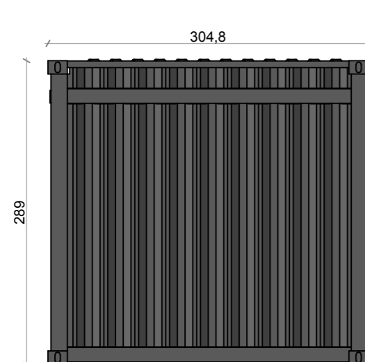
POSTERIOR
