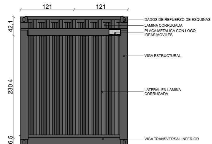
LATERAL DERECHO
