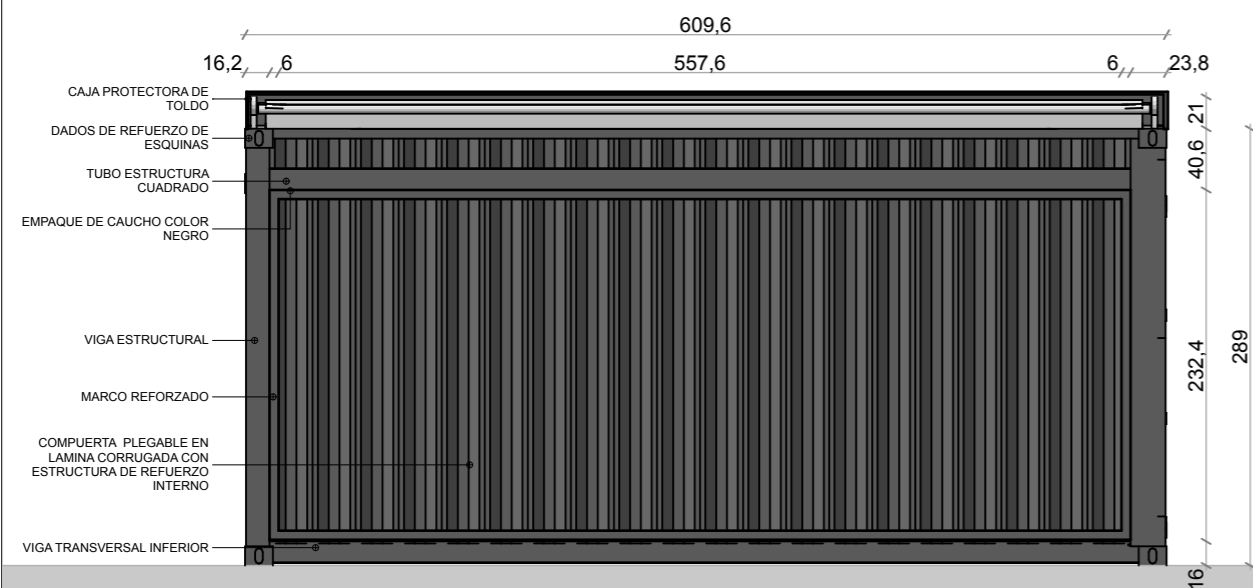
ALZADO
